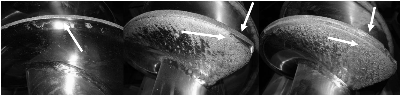
Abb. 13-15: Indizes für die Notwendigkeit der Schneckenaufarbeitung
