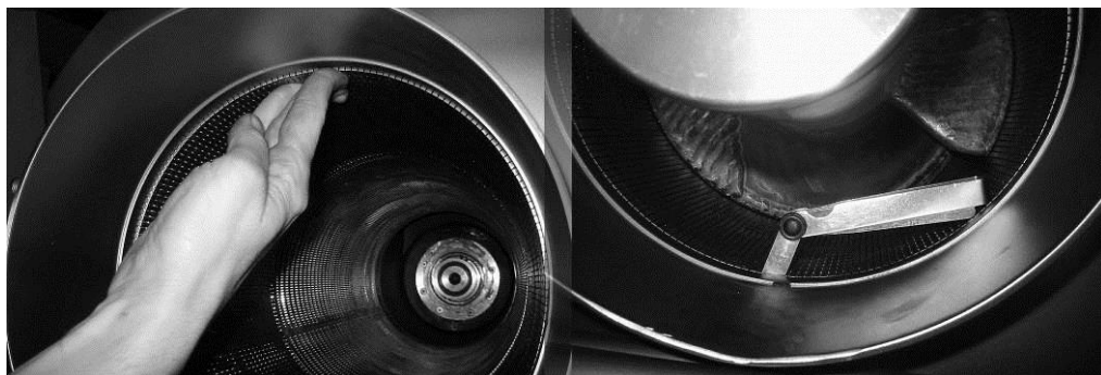
Abb.13-10: Bewegliches Sieb im Separator, Prüfung der Schwimmfähigkeit mit der Hand (links)
