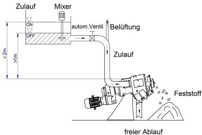
Abb.4-6 Beschickung über die Schwerkraft durch einen höher gelegenen Tank
