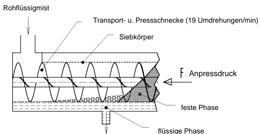
Abb. 3-1 Funktionsbeschreibung
