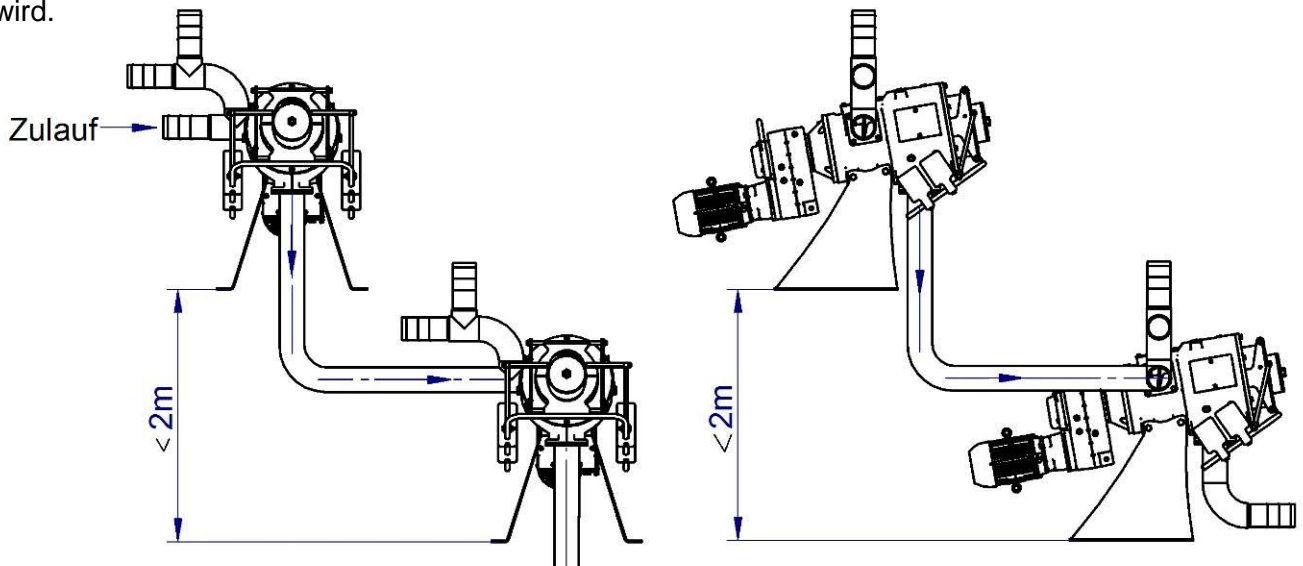
Abb. 10-1 Typische Anordnung zum Betrieb von 2 Separatoren in Reihenschaltung
