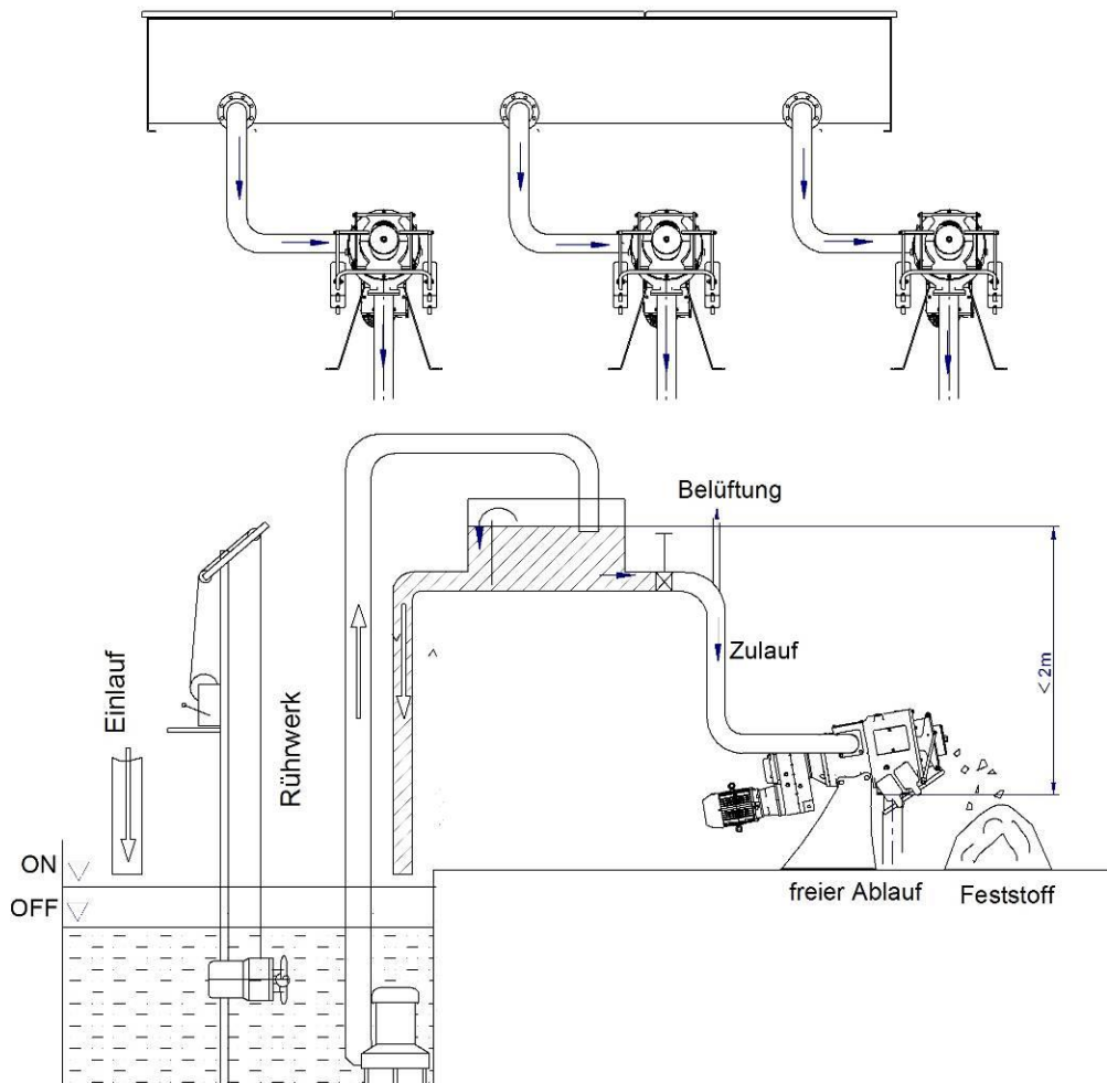
Abb 9-1. Typische Anordnung zum Betrieb von 3 Separatoren in Parallelschaltung
