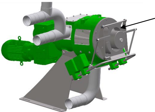
Abb. 7-2 Ausbringklappen
