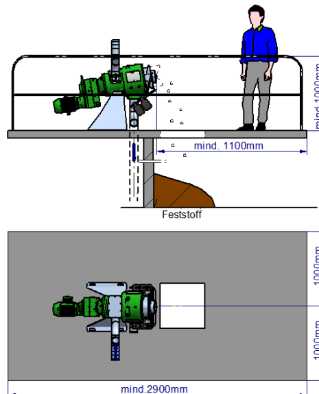
Abb. 4-4 Dimensionierung Aufstellplatz
