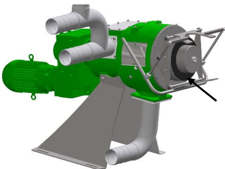
Abb. 7-3 Stopfenbildungshilfe
