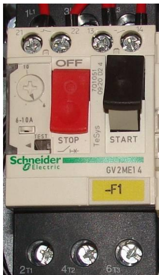
Abb. 15-3 Motorschutz F1
