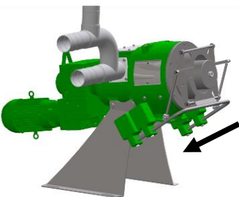
Abb. 7-5 Stopfen zu weich
