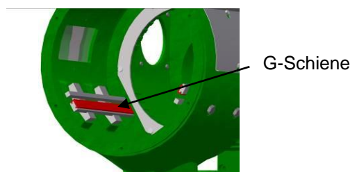
Abb. 13-5 Gehäuse Separator Compact mit Siebführungsschienen und G-Kunststoffprofilschienen
