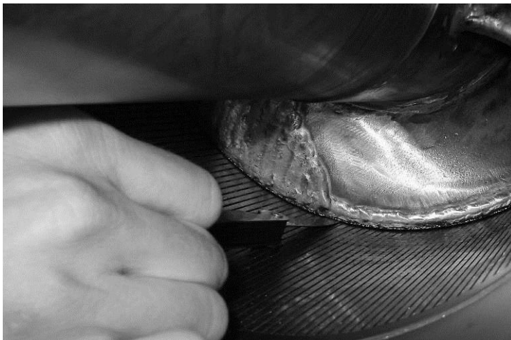
Abb. 13-14: Messung des Arbeitsspalt zwischen Sieb und Schnecke, gemessen wird an der Unterseite des Siebes bei Stillstand der Maschine, die Messung ergibt den 2-fachen Arbeitsspalt, da im ruhenden Zustand das Sieb oben auf der Schnecke aufliegt.
