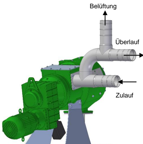
Abb.4-7 Einlauf-Aufbau
