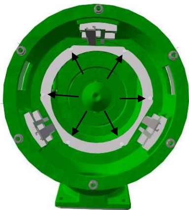
Abb. 13-7 Verschleißring
