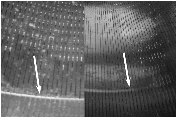
Abb.13-8 : Verschleiß im Sieb durch verspanntes Sieb (links)
