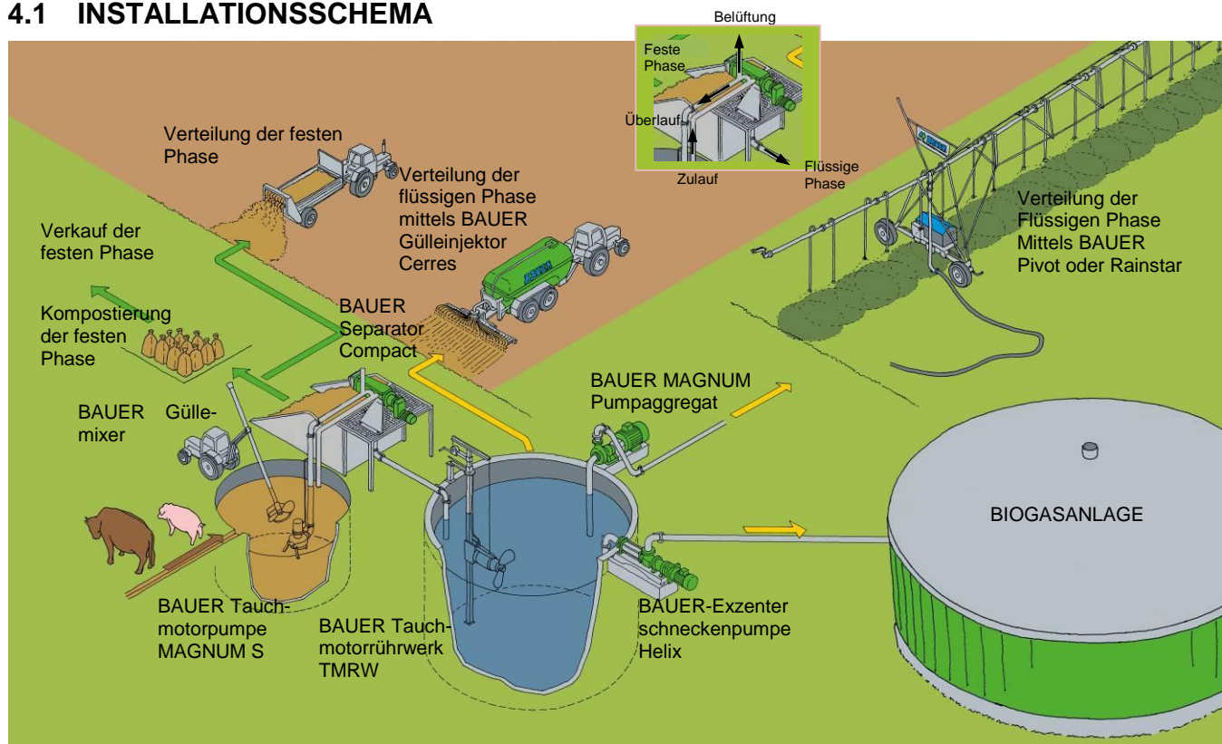
Abb. 4-1 Installationsschema
