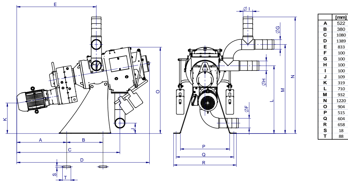
Abb. 4-3 Abmessungen Separator Compact
