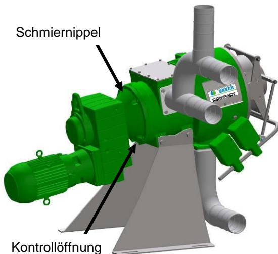
Abb. 13-1 Versorgung mit Sperrmedium
