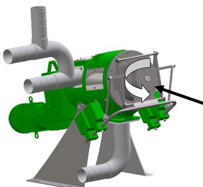
Abb. 5-1 Drehrichtung Schnecke
