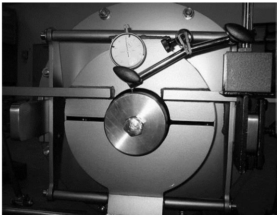
Abb. 13-12: Kontrolle des Taumelschlags der Schnecke
