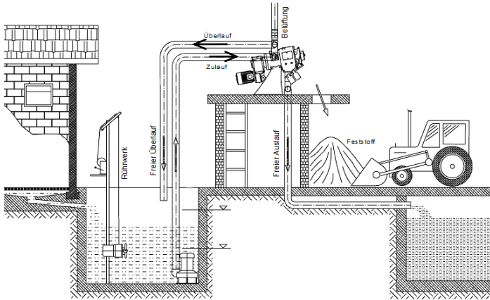
Abb.4-5 Beschickung über Pumpe
